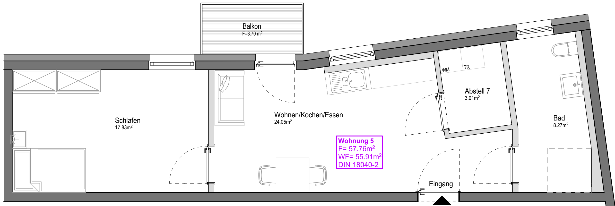
Grundriss Wohnung 5 (1.0G)
